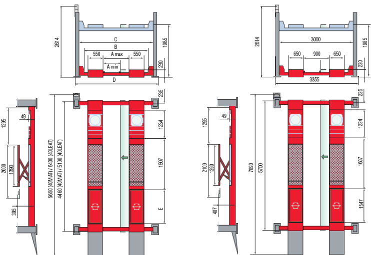
PROLIFT 440LEAT
